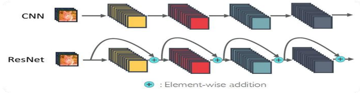
Şekil 4: CNN ve ResNet mimarilerinin karşılaştırılması (Ultralytics, 2026)
