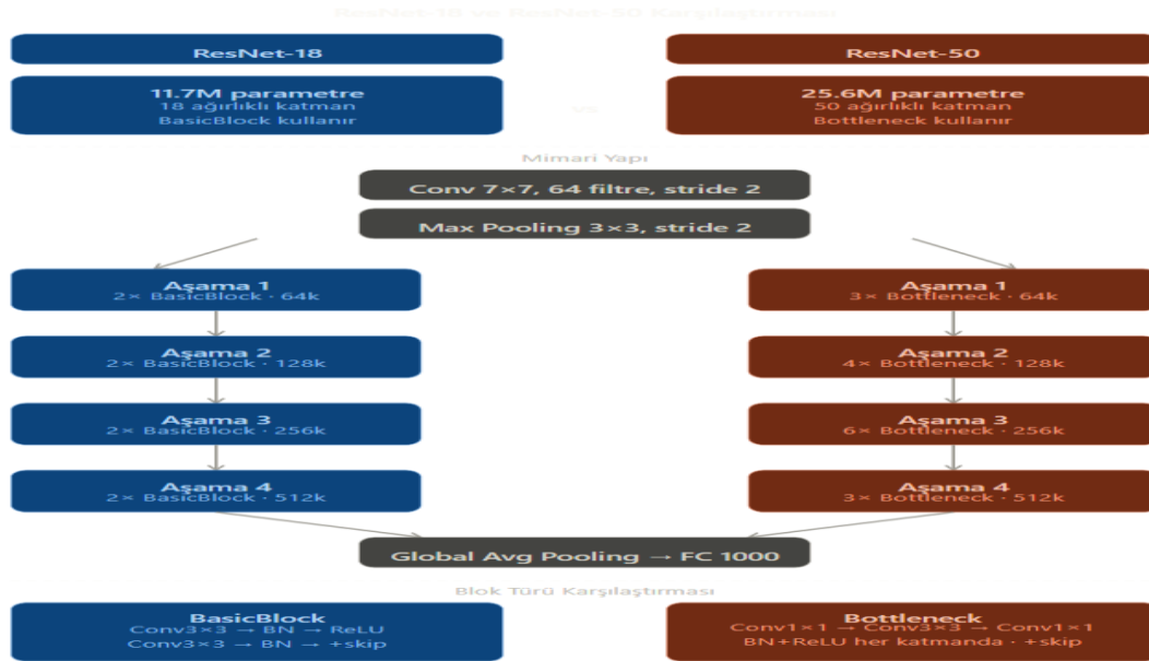
Şekil 5: ResNet-18 ve ResNet-50 mimarilerinin karşılaştırılması
