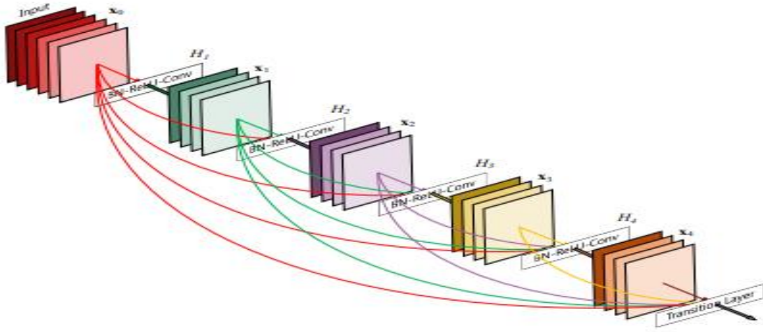
Şekil 6: DenseNet model mimarisi
