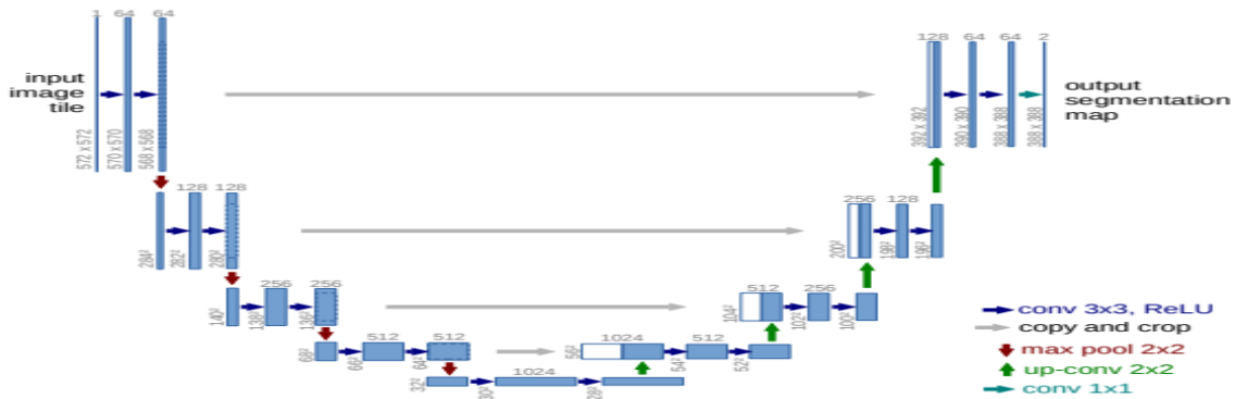
Şekil 3: U-Net model yapısı
